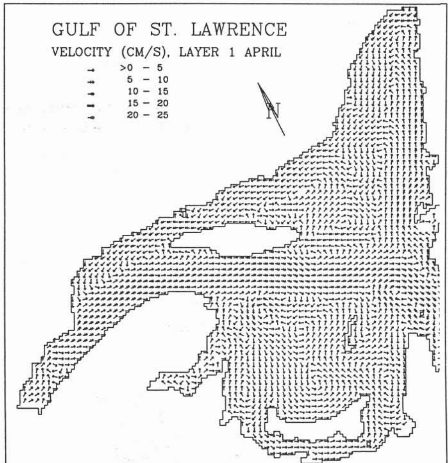
Circulation à la surface du Golfe du Saint-Laurent, en avril
