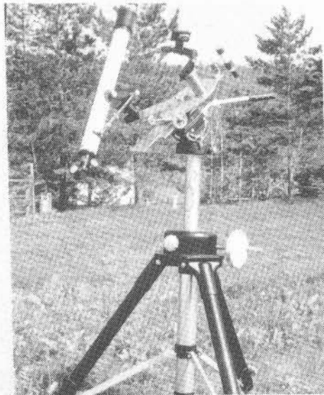
Cet instrument de travail, nommé «table équatoriale polaire», a été réalisé et construit manuellement par Sylvain Levesque. Les principales pièces sont en cuivre. L'appareil sert à faire de la photographie de l'espace (astrophotographie).
