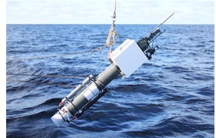
Flotteur Argo, IOW/M. Naumann
